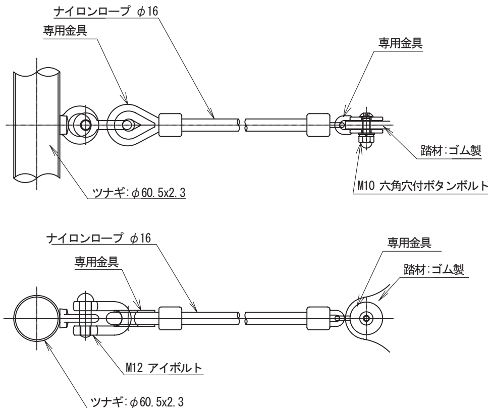
ロープ部取合詳細図 1:5
