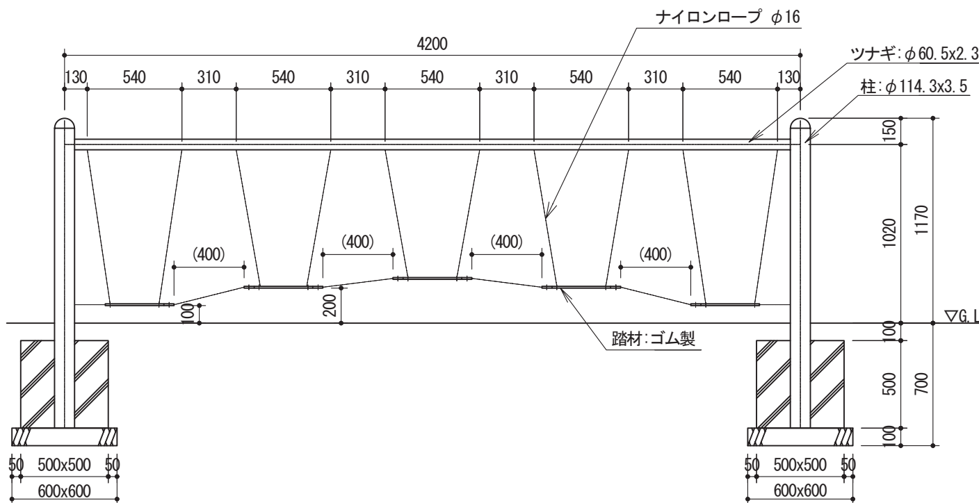
立面図 1:30
