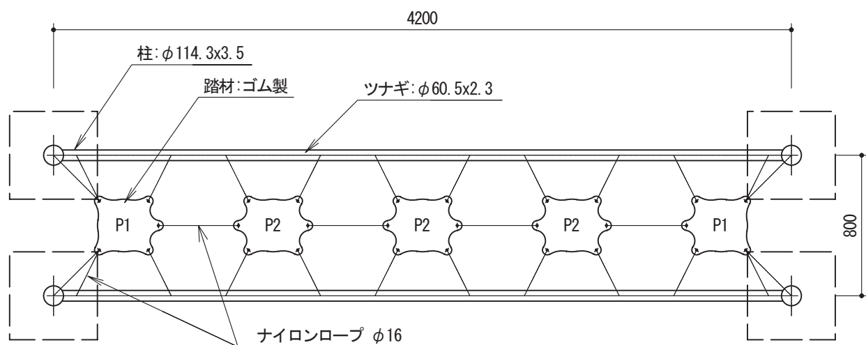
立面図 1:30
