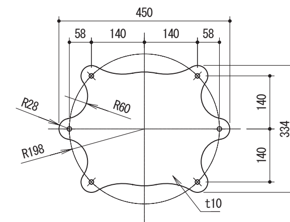
P2踏材詳細図 1:10
