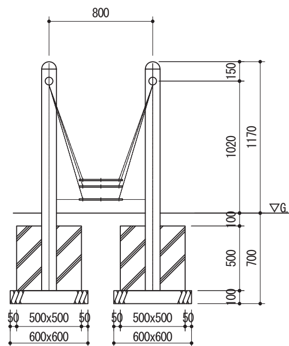
立面図 1:30
