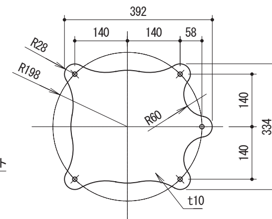
P1踏材詳細図 1:10
