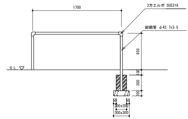
安全柵立面図 1 : 30
